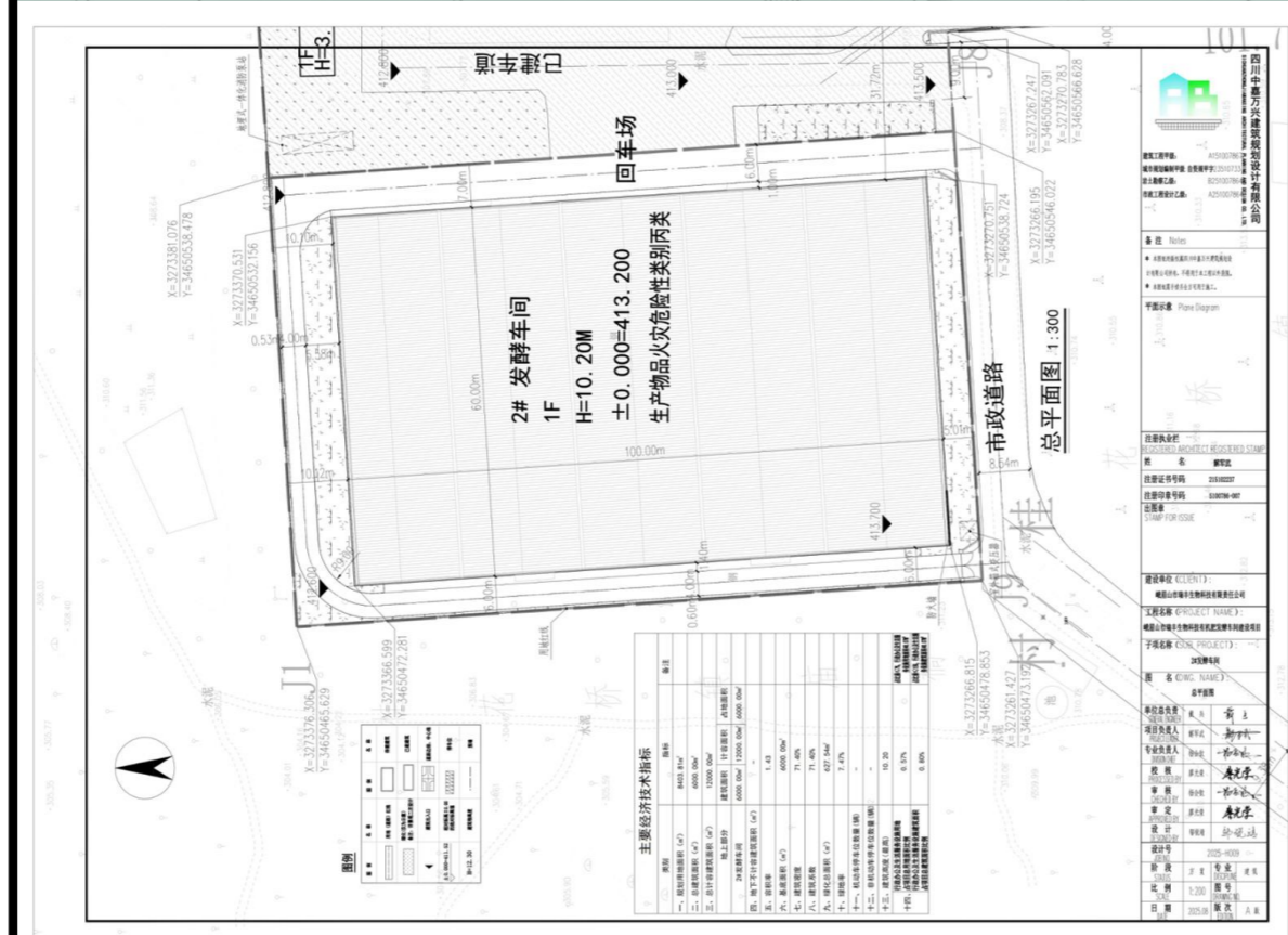
总平面图
