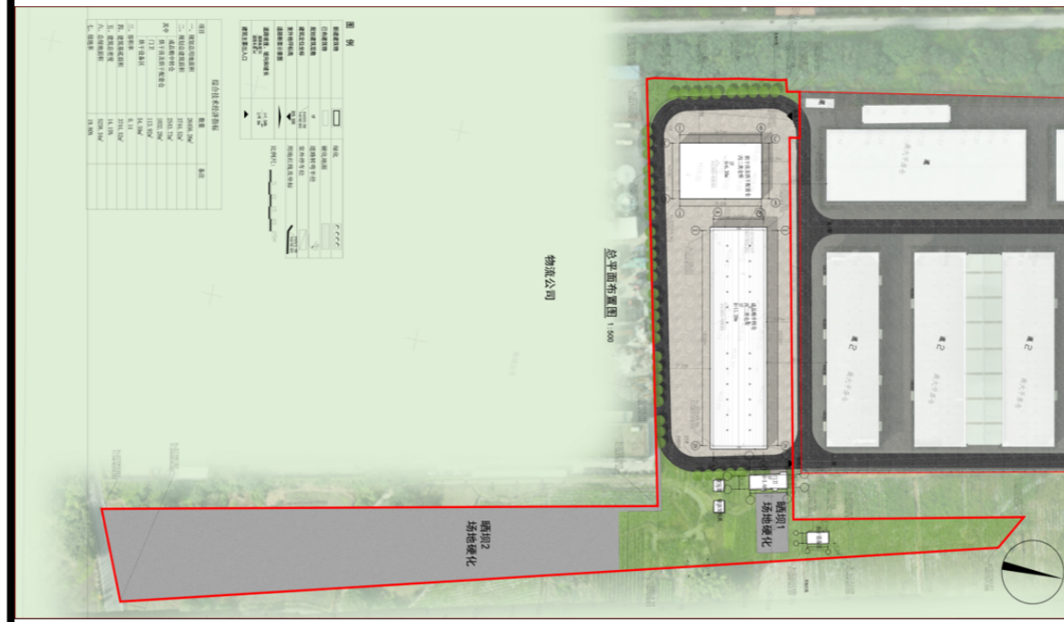
总平面图
