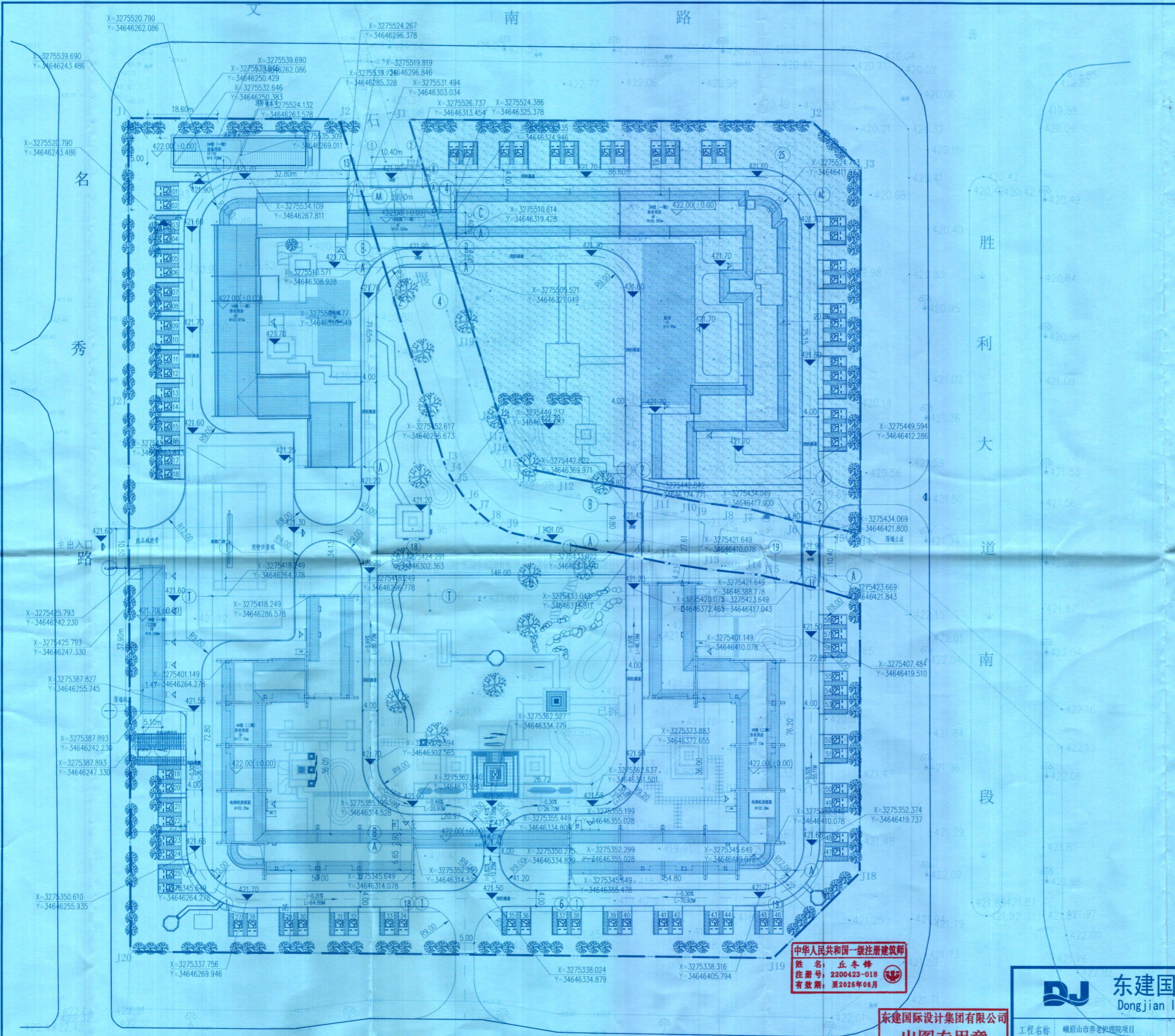
总平面图 1:500 秀湖大道
